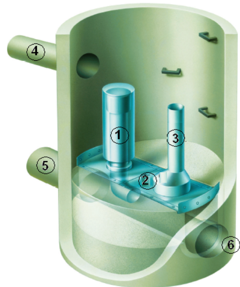
HydroFlush installeret i en regnvandsbrønd med spildevandsgennemløb
